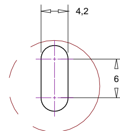
Szczegół A Skala 2:1
