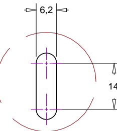
Szczegół A Skala 1:1
